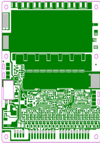
顶层走线图
