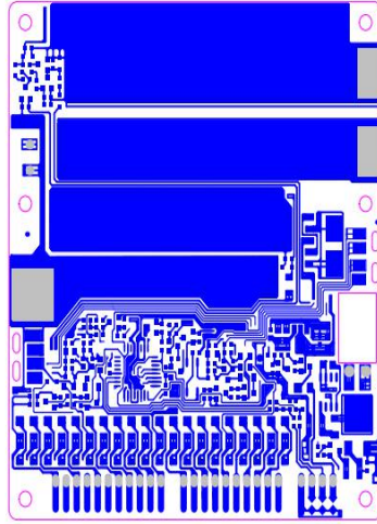
底层走线图
