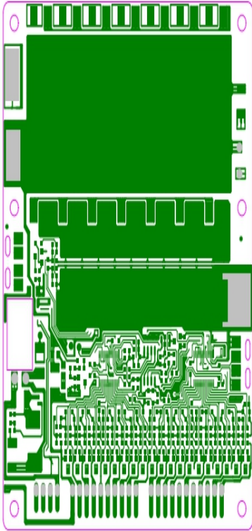
顶层走线图
