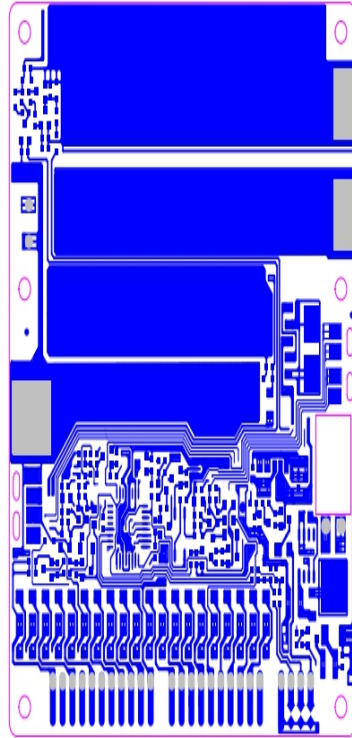
底层走线图
